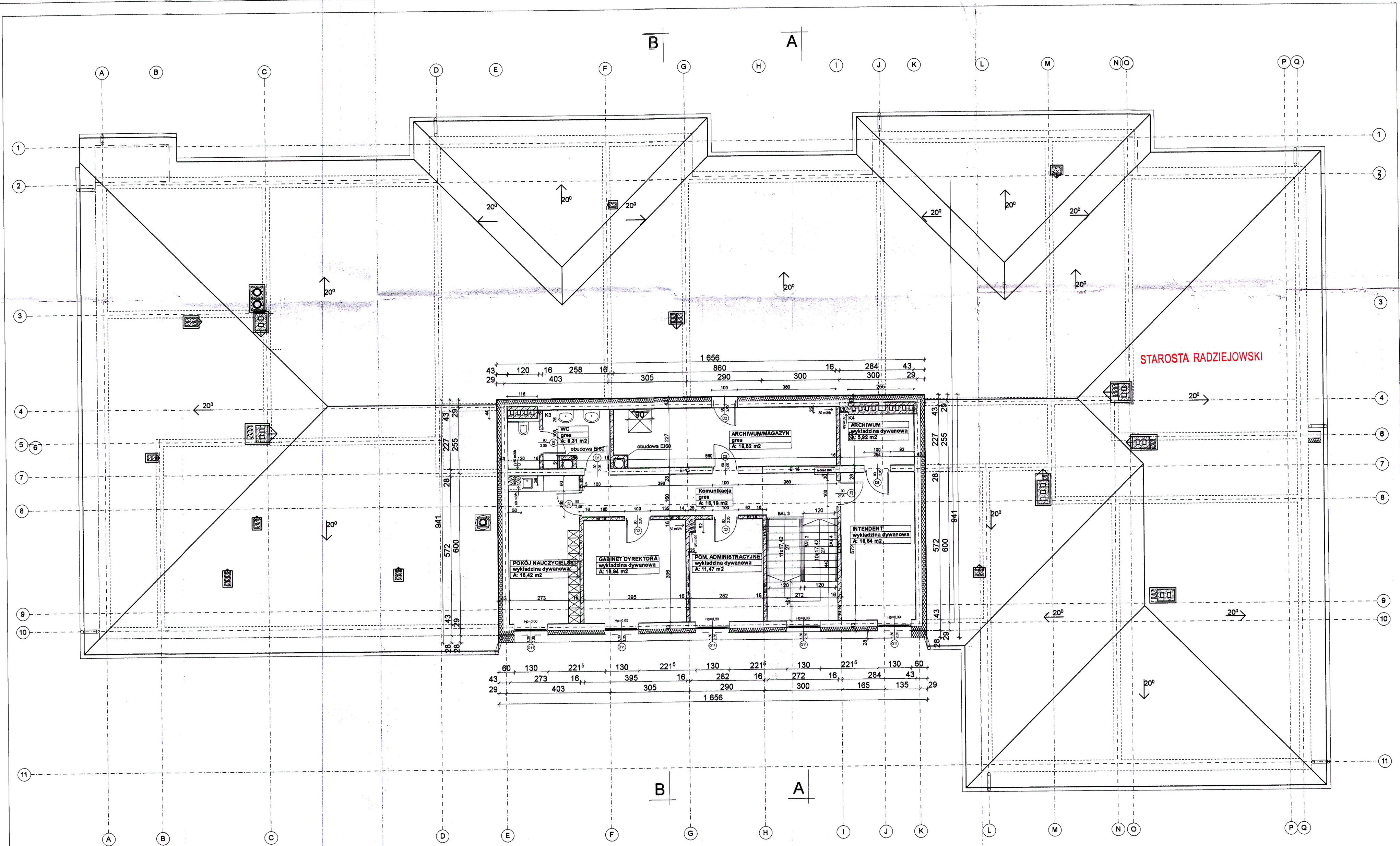
RZUT PIĘTRA 1: 100
