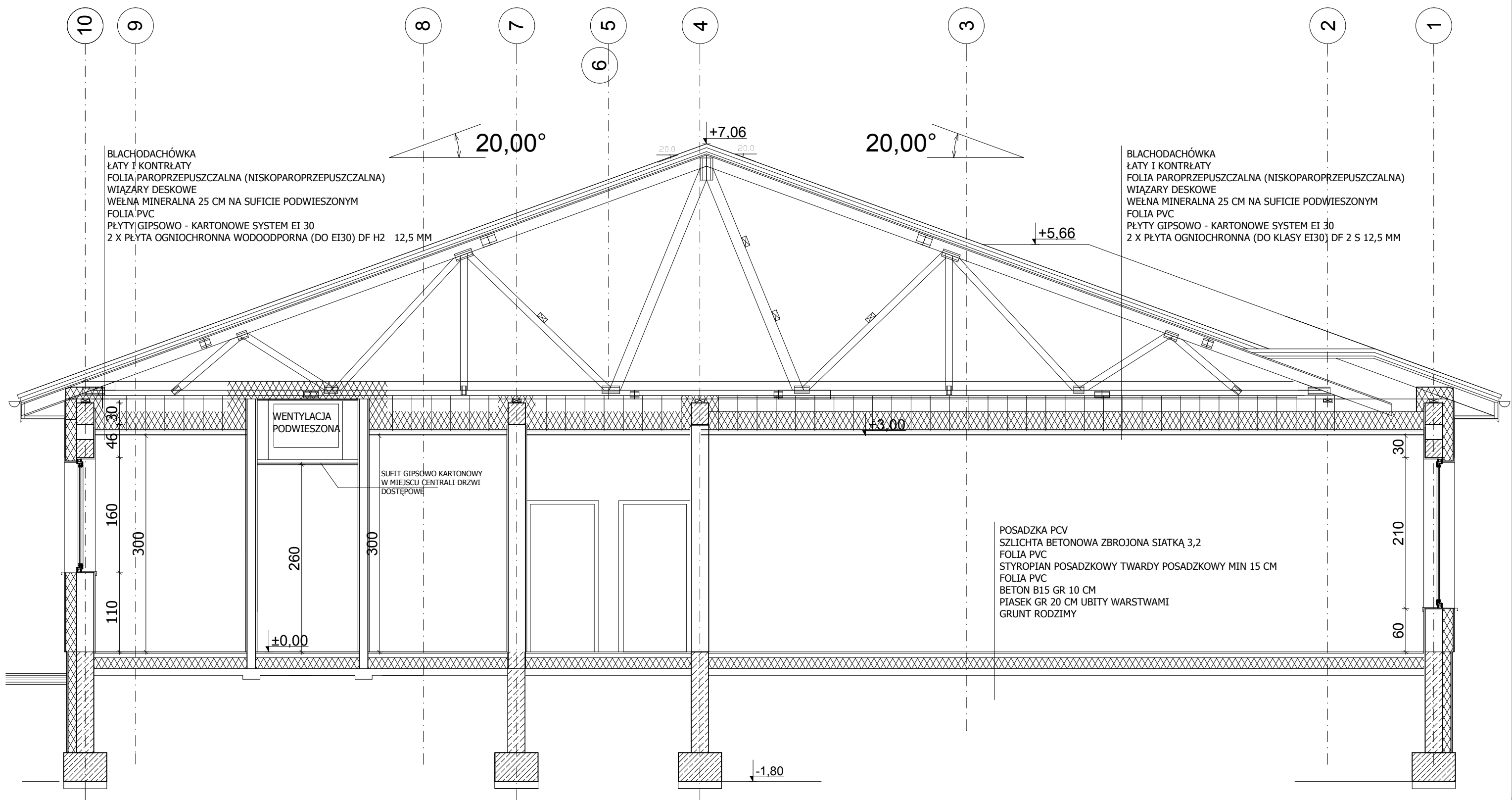
PRZEKRÓJ D- D 1: 50
