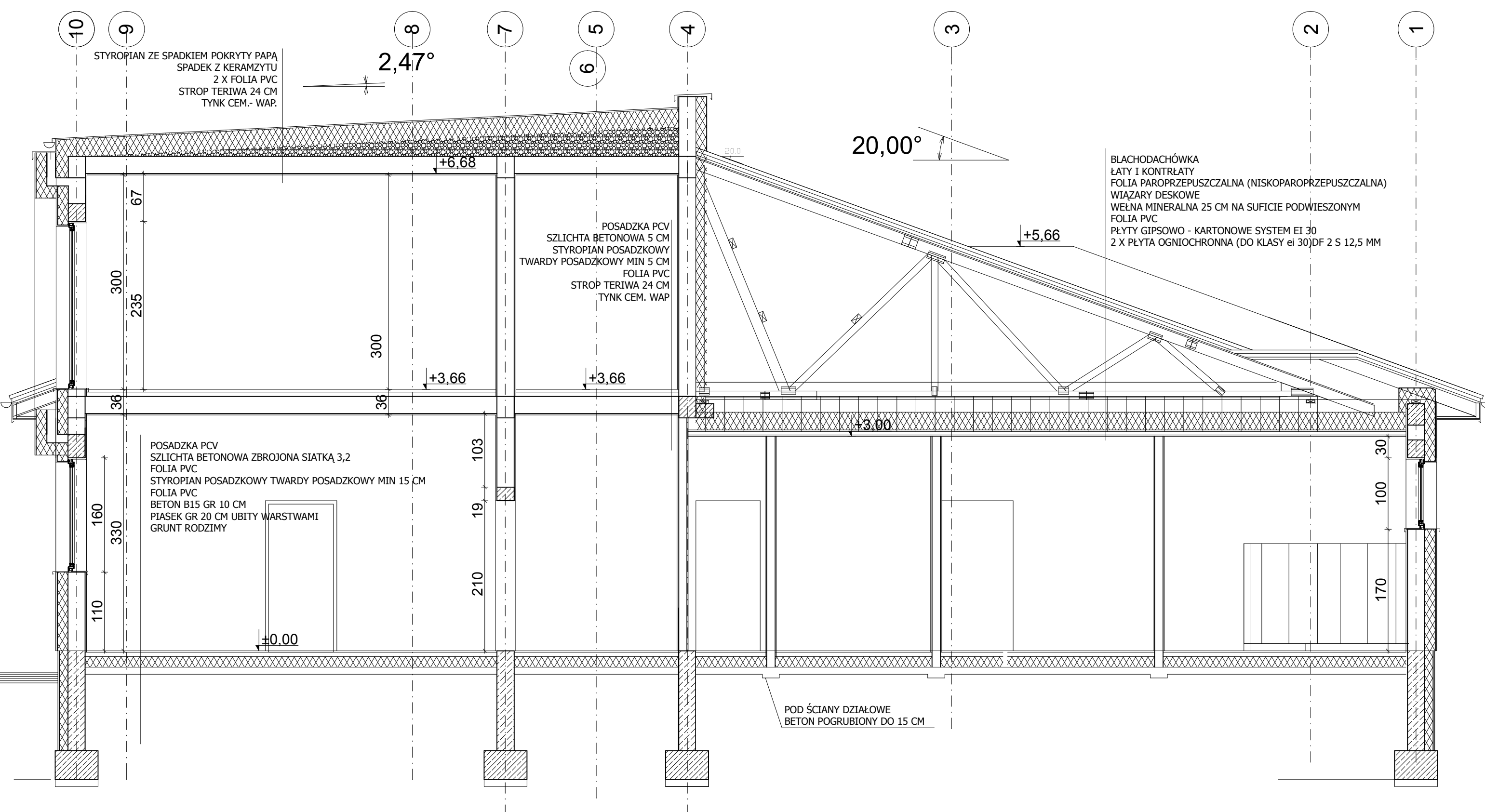
PRZEKRÓJ B- B 1: 50
