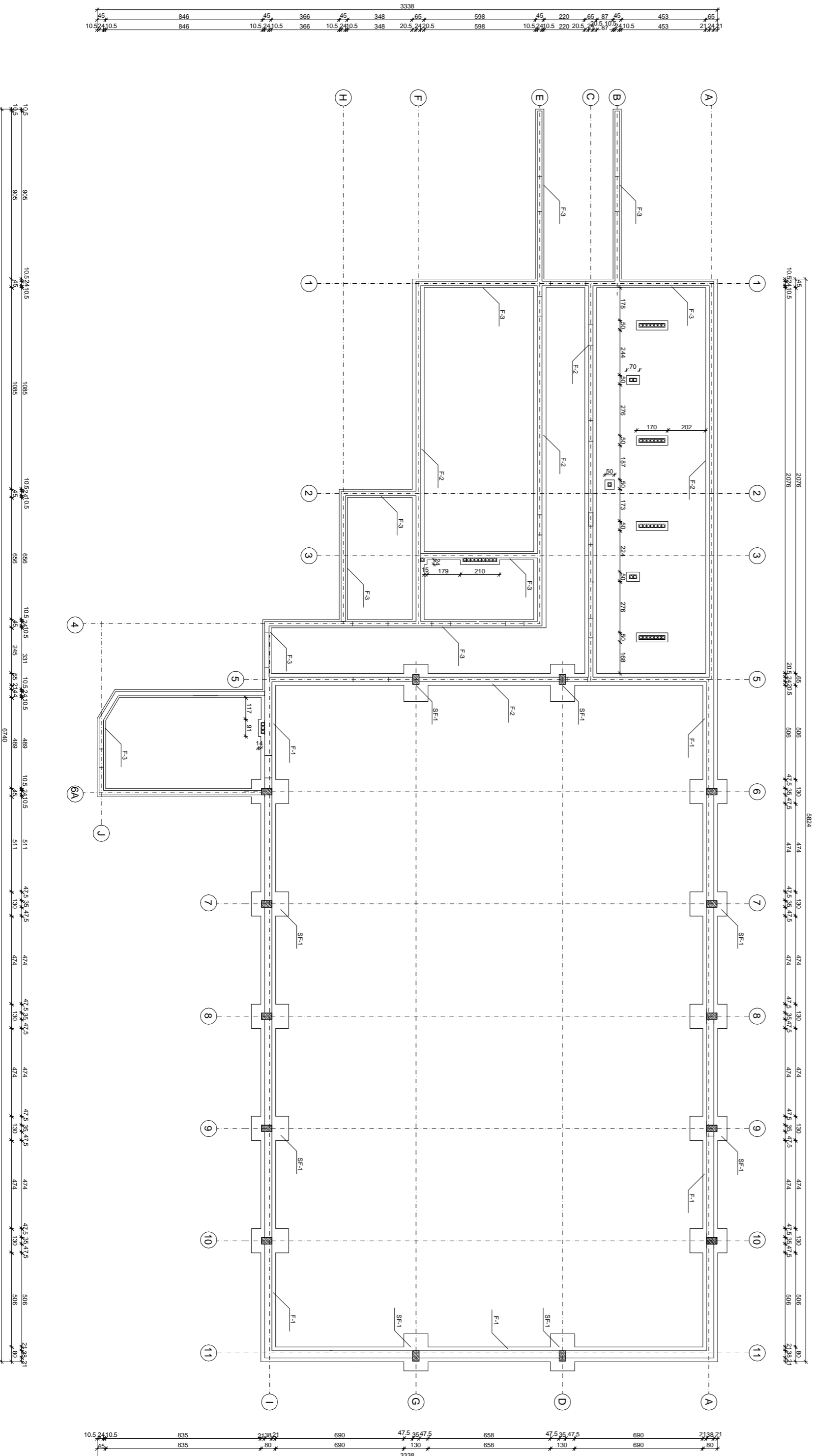
RZUT FUNDAMENTOW Skala 1:100
