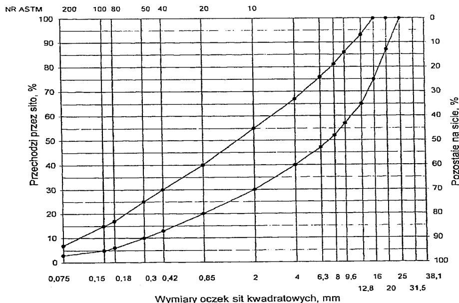
Rys. 7. Krzywe graniczne uziarnienia mieszanki mineralnej BA od 0 do 20 mm do warstwy wiążącej, wyrównawczej i wzmacniającej nawierzchni drogi o obciążeniu ruchem KR1 lub KR2
