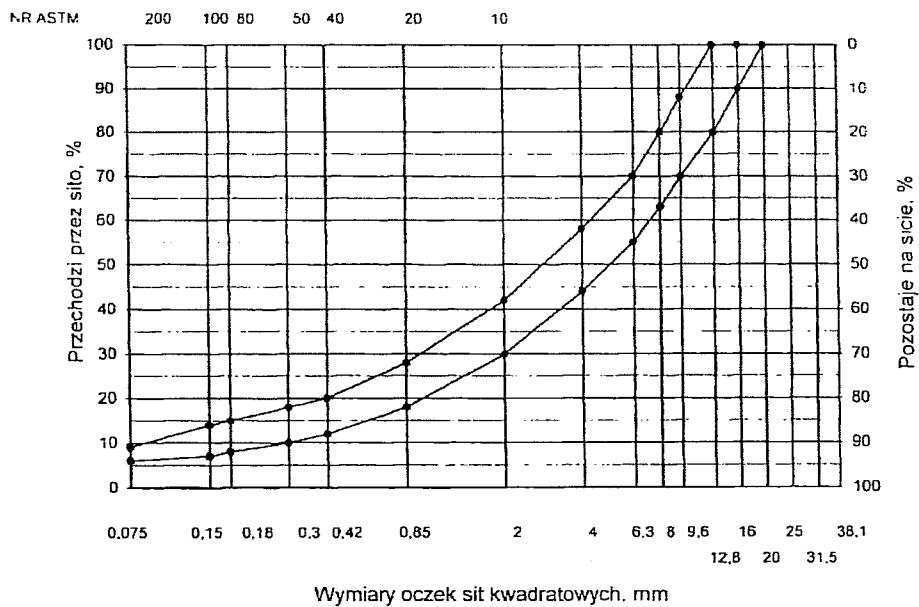
Rys. 5. Krzywe graniczne uziarnienia mieszanki mineralnej BA od 0 do 16 mm do warstwy ścieralnej nawierzchni drogi o obciążeniu ruchem od KR3 do KR6
