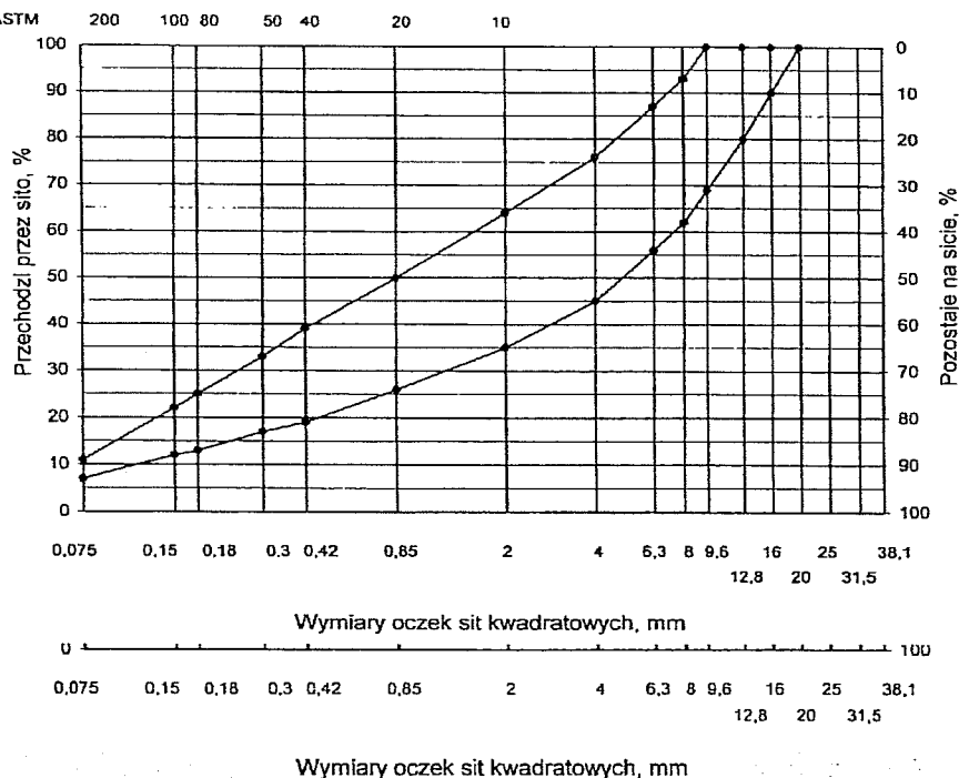
Rys. 1. Krzywe graniczne uziarnienia mieszanki mineralnej BA od 0 do 20 mm do warstwy ścieralnej nawierzchni drogi o obciążeniu ruchem dla KR1 lub KR2
