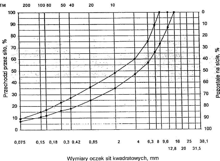
Rys. 6. Krzywe graniczne uziarnienia mieszanki mineralnej BA od 0 do 12,8 mm do warstwy ścieralnej nawierzchni drogi o obciążeniu ruchem od KR3 do KR6
