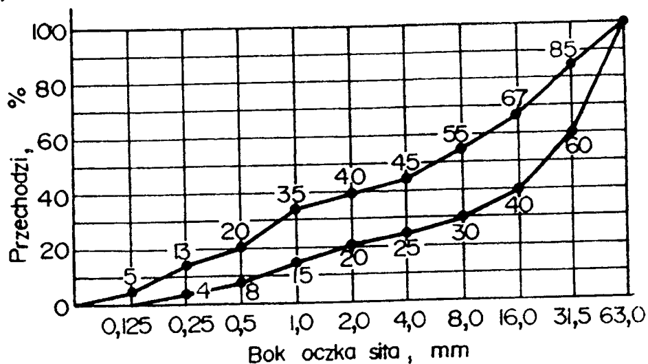
Rysunek 2. Graniczne krzywe uziarnienia kruszywa do betonu C 8/10 od 0 do 63 mm.
