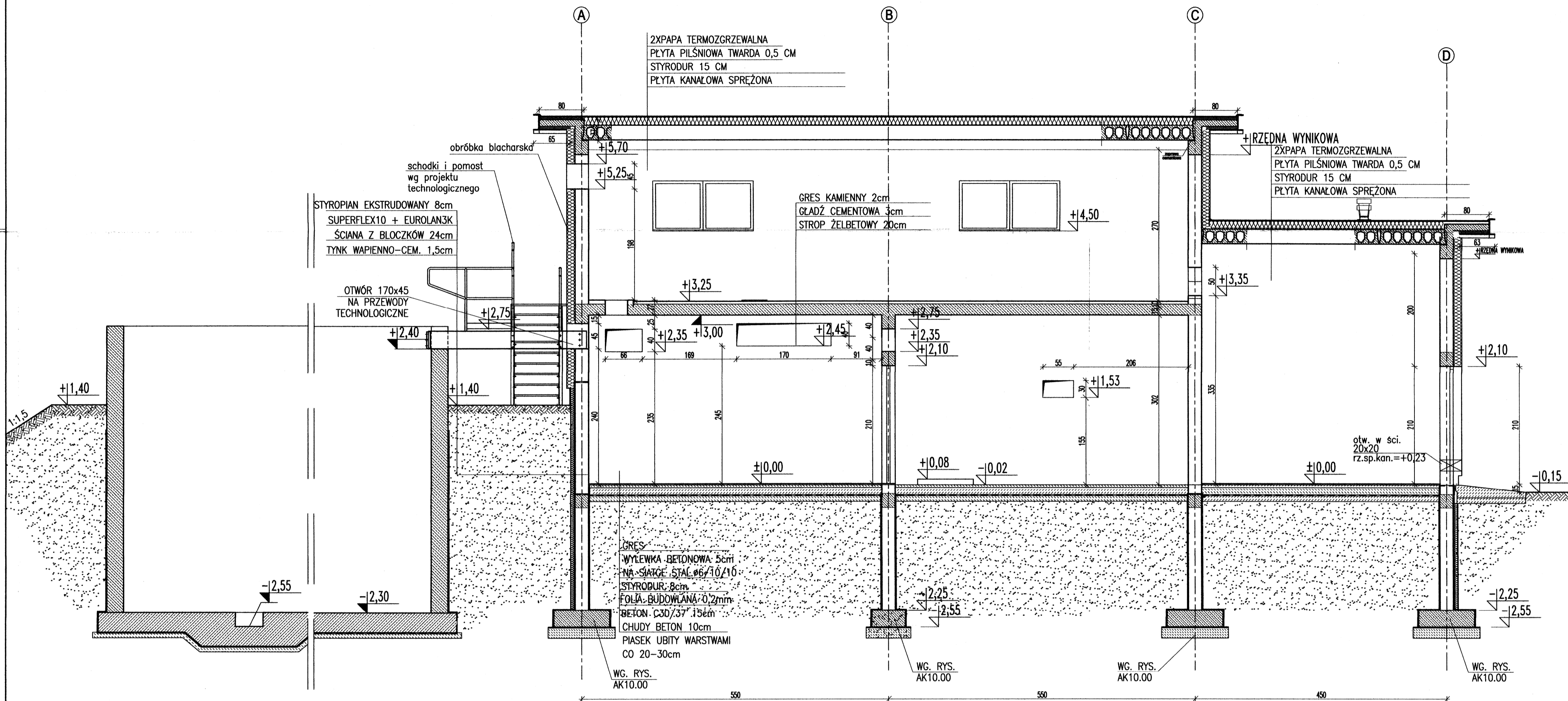
PRZEKRÓJ I-I 1:50
