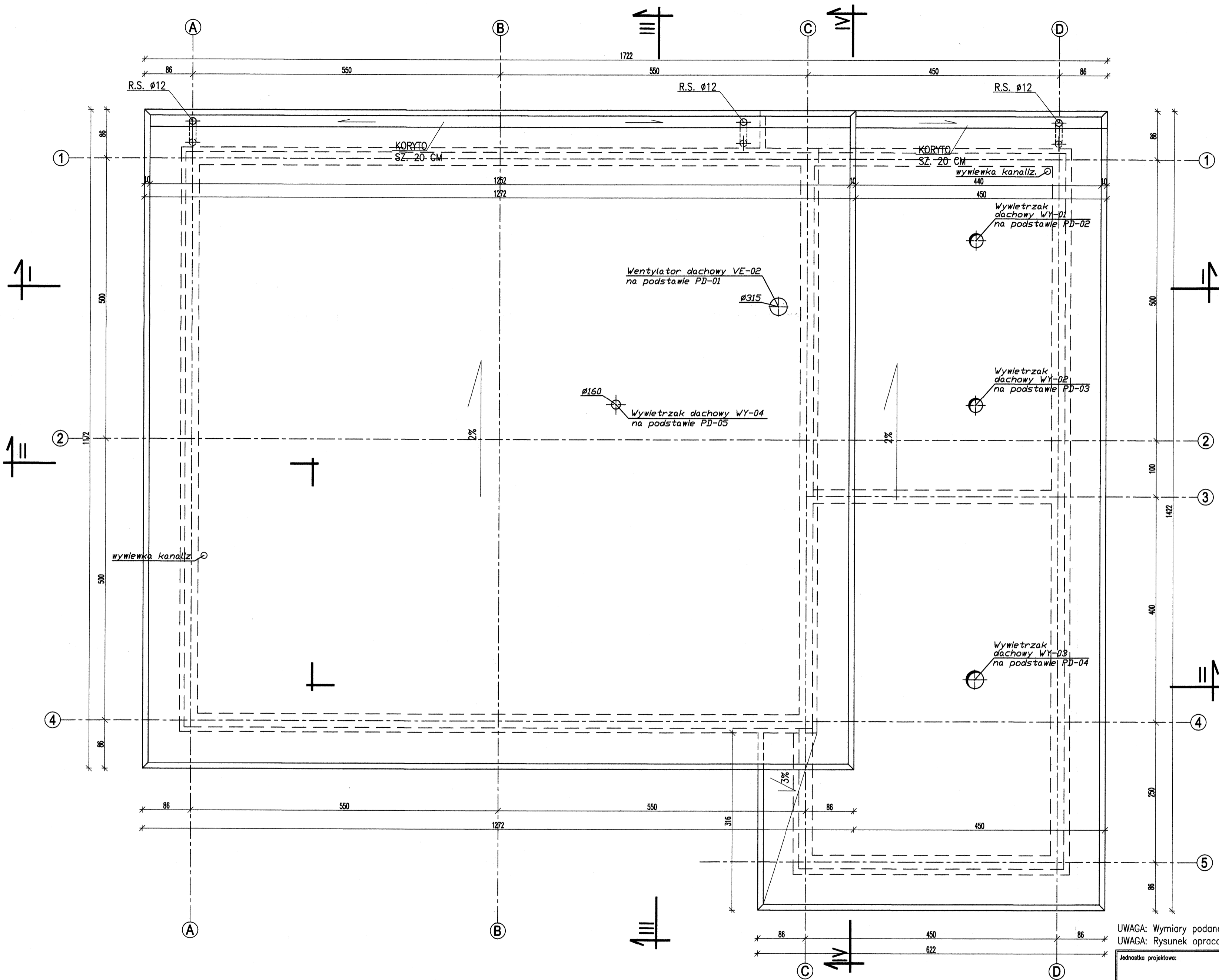
RZUT POŁACI DACHOWYCH 1:50
